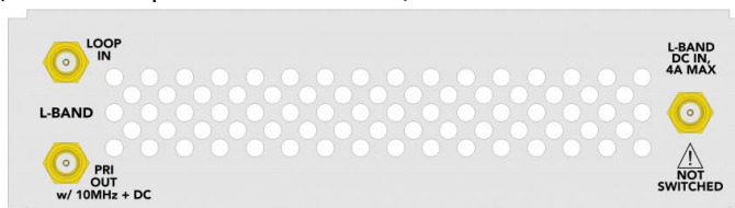
Рисунок 8. Модуль SMD 940
