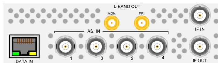
Рисунок 6. Модуль SMD 920 в комбинации с модулем SMD 910
