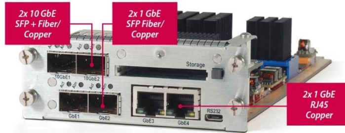
Оptionальный модуль Quad GbE I/O в ProStream™ 9100 для обработки до 2 Gb трафика.
